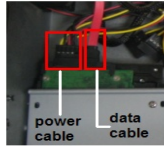
Рис. 1.1.4. Подключение HDD
