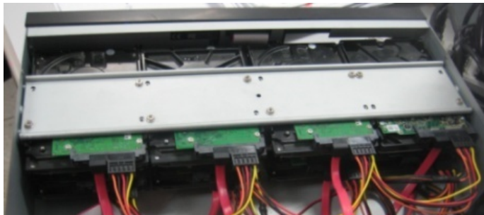
Рис. 1.1.7. Установка HDD
